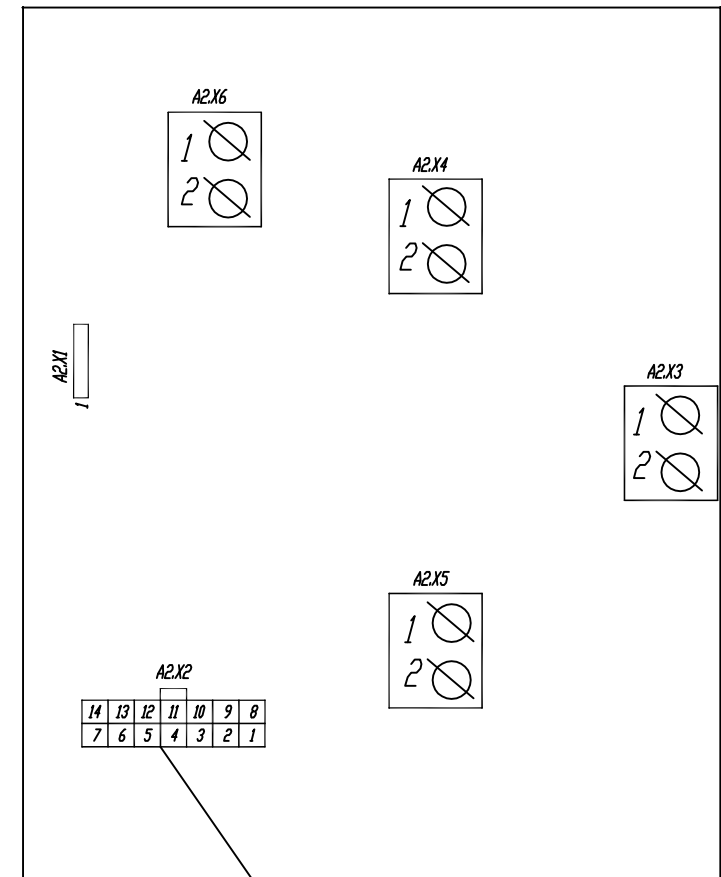
Вид со стороны проводов розетки.
